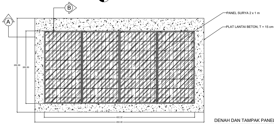
DENAH DAN TAMPAK PANEL SURYA
