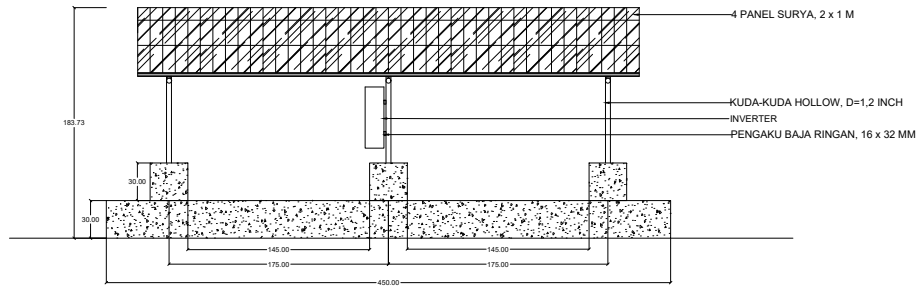
TAMPAK DEPAN PANEL SKALA 1:30
